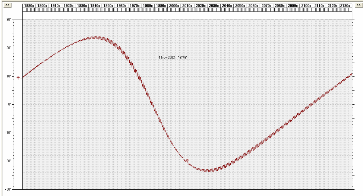
Afbeelding declinatie Pluto 1890 tot 2130. In 1940 zie je een keerpunt van Pluto in het noordelijk halfrond en anno 2012 staan we weer voor een keerpunt van Pluto, maar dan in het zuidelijk halfrond.
